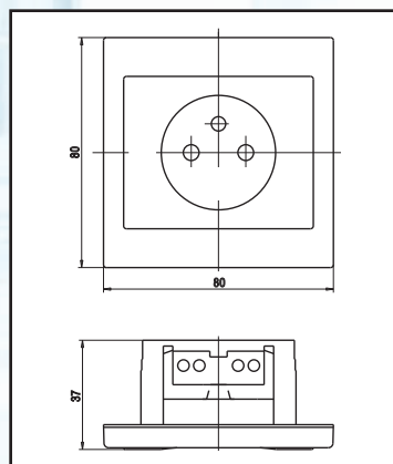
Zásuvka PRAKTIK 4 FN 150 65
