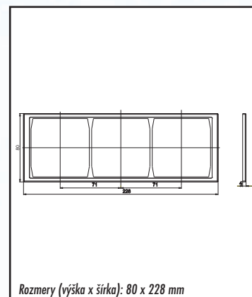
Trojrámček PRAKTIK 4 FA 127 43
