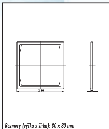
Jednorámček PRAKTIK 4 FA 127 41
