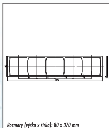
Päťrámček PRAKTIK 4 FA 127 45
