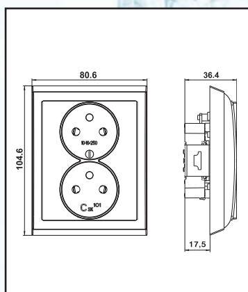
Dvozásuvka PRAKTIK 4 FN 150 66
