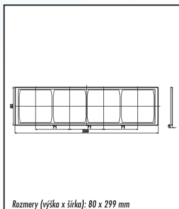
Štvorrámček PRAKTIK 4 FA 127 44
