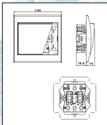
Vypínač PRAKTIK 4 FN 580 00
