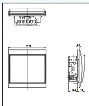
Vypínač PRAKTIK výstavba 4 FN 580 100
