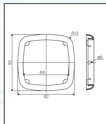
Jednorámček MODUL 4 FA 127 27
