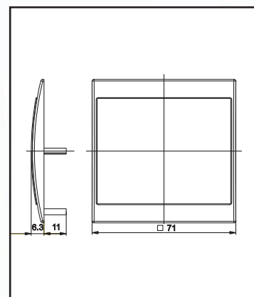
Zaslepovací kryt do rámečkov PRAKTIK 4 FA 261 51
