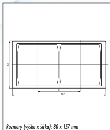
Dvojrámček PRAKTIK 4 FA 127 42
