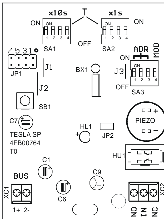
Obr. 1. Pripojné a nastavovacie miesta spínacieho modulu 2-BUS 4 FN 230 30
